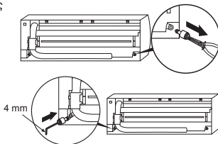
Σωλήνας αποστράγγισης
