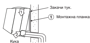
Кука
