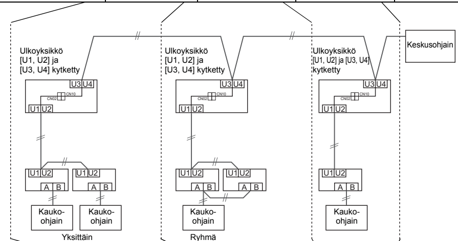
Sisäyksiköt (automaattinen asetus)
