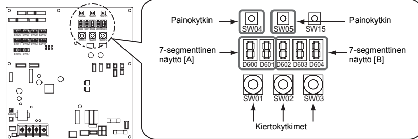
Käyttöliittymän PC-levy
