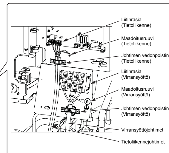
Sähköisen ohjausrasian suojus
