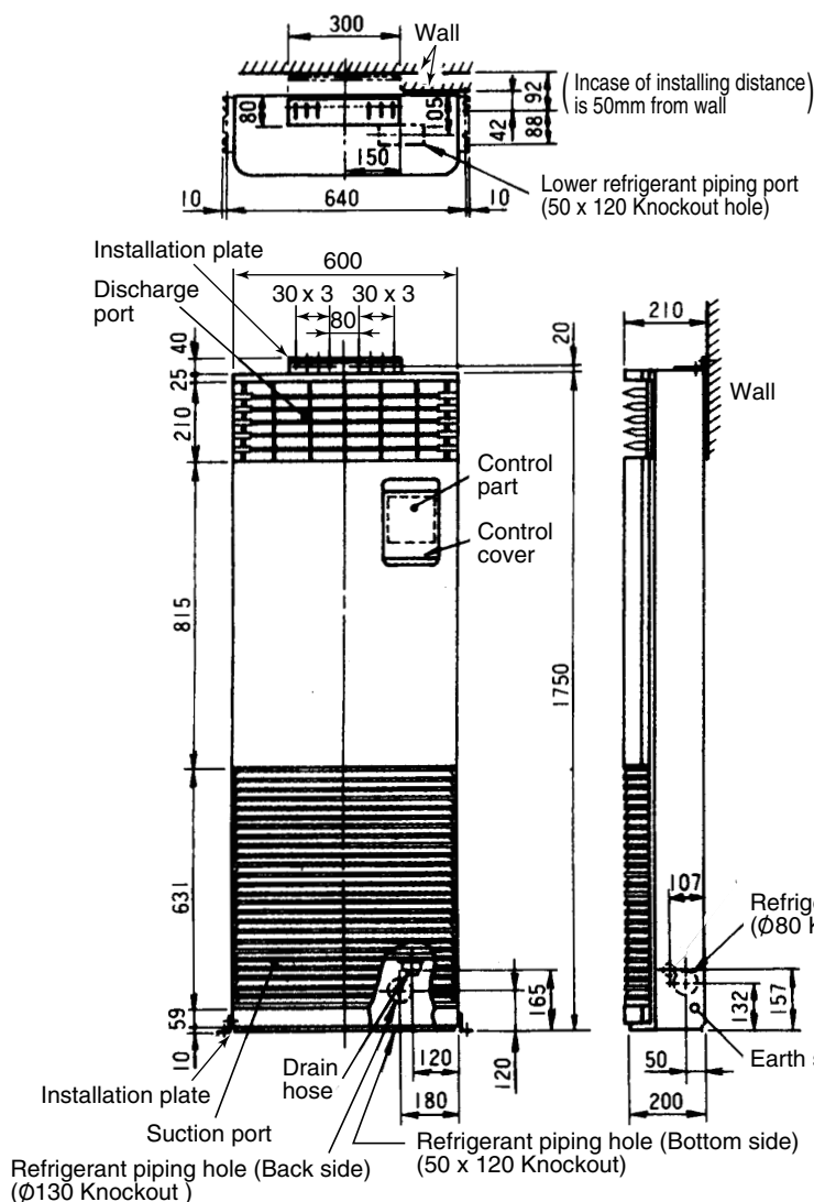
Dimensions
