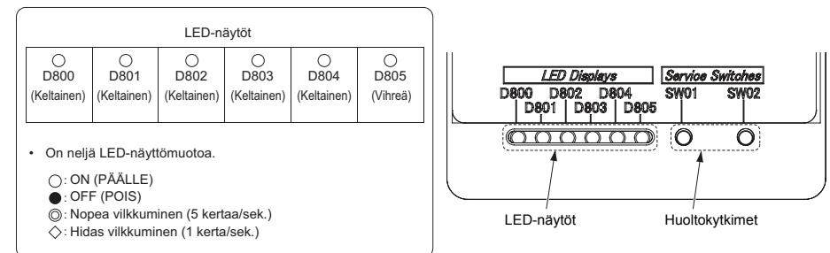
LED-näytön oletustila
